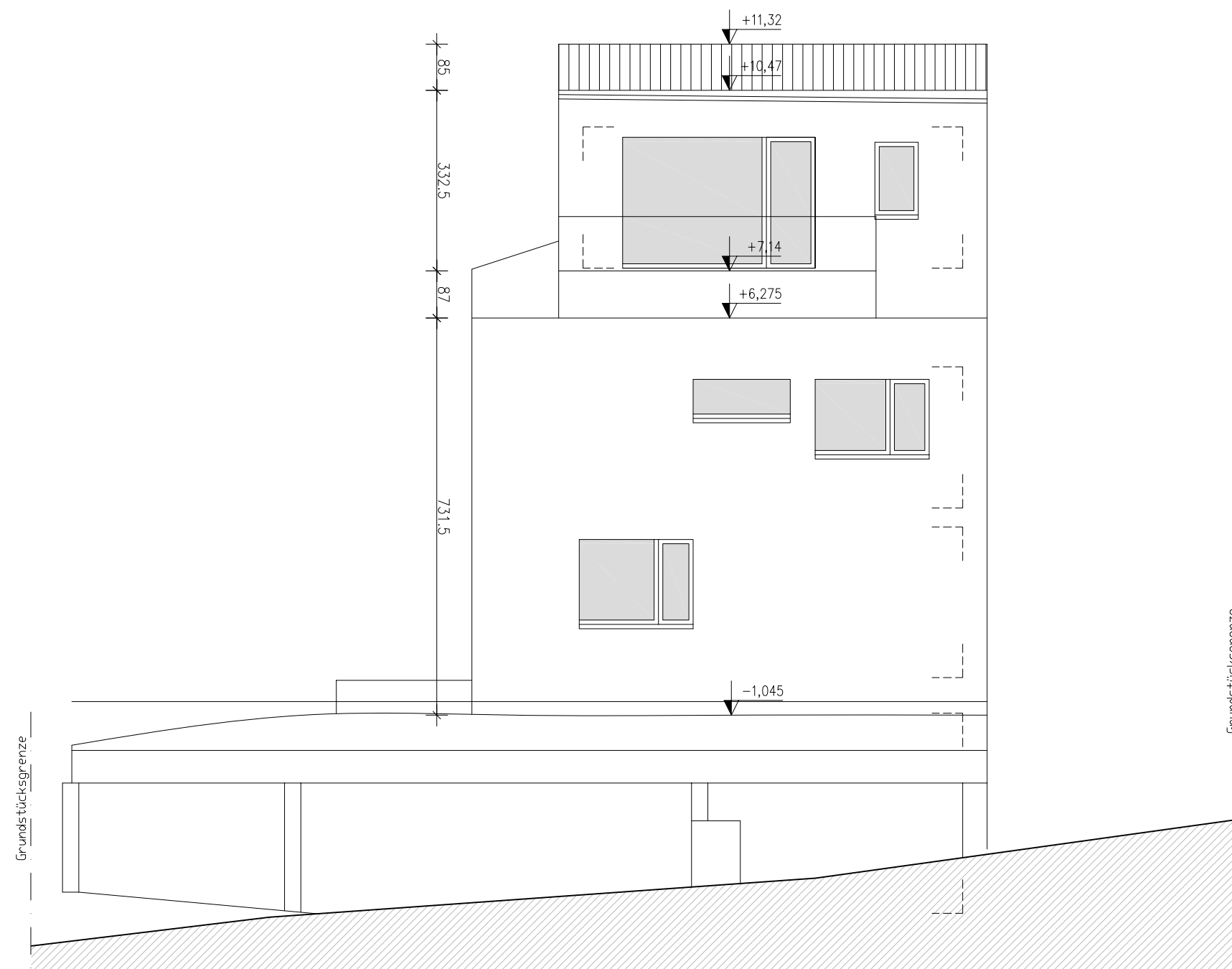
NORDOSTFASSADE
