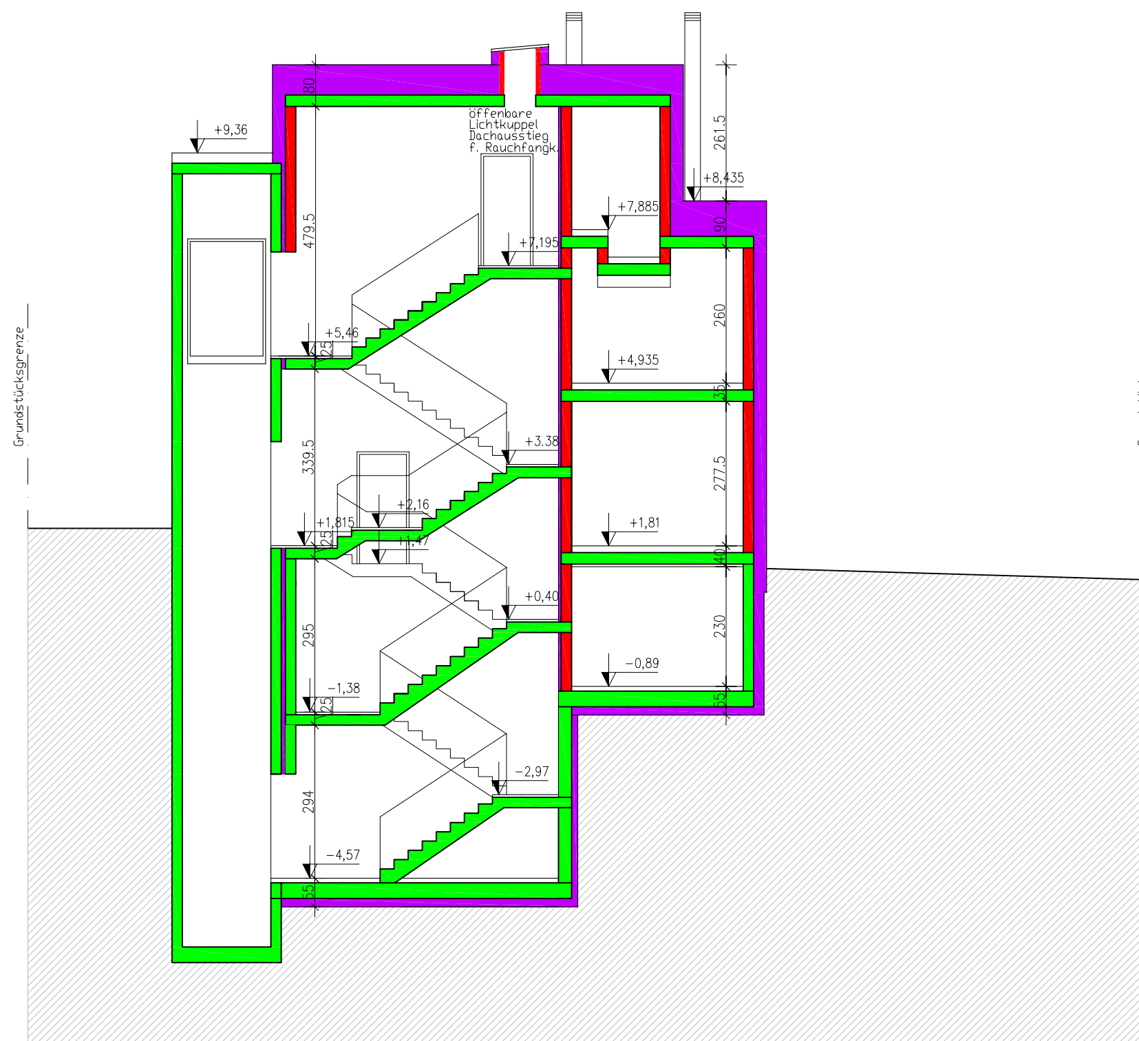
SCHNITT AA
