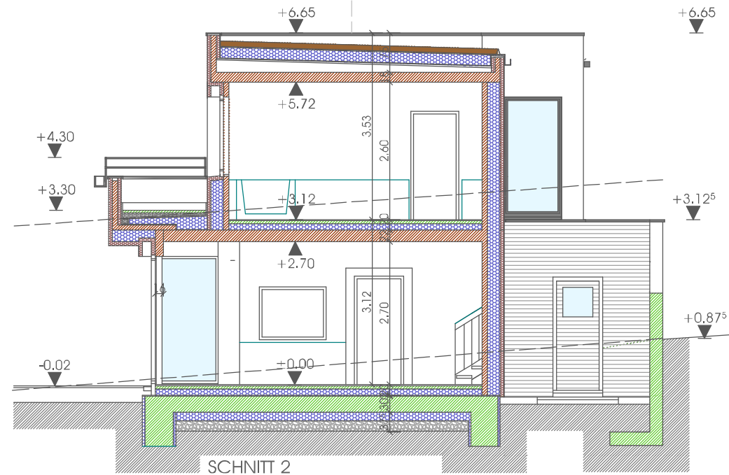
SCHNITT 2
