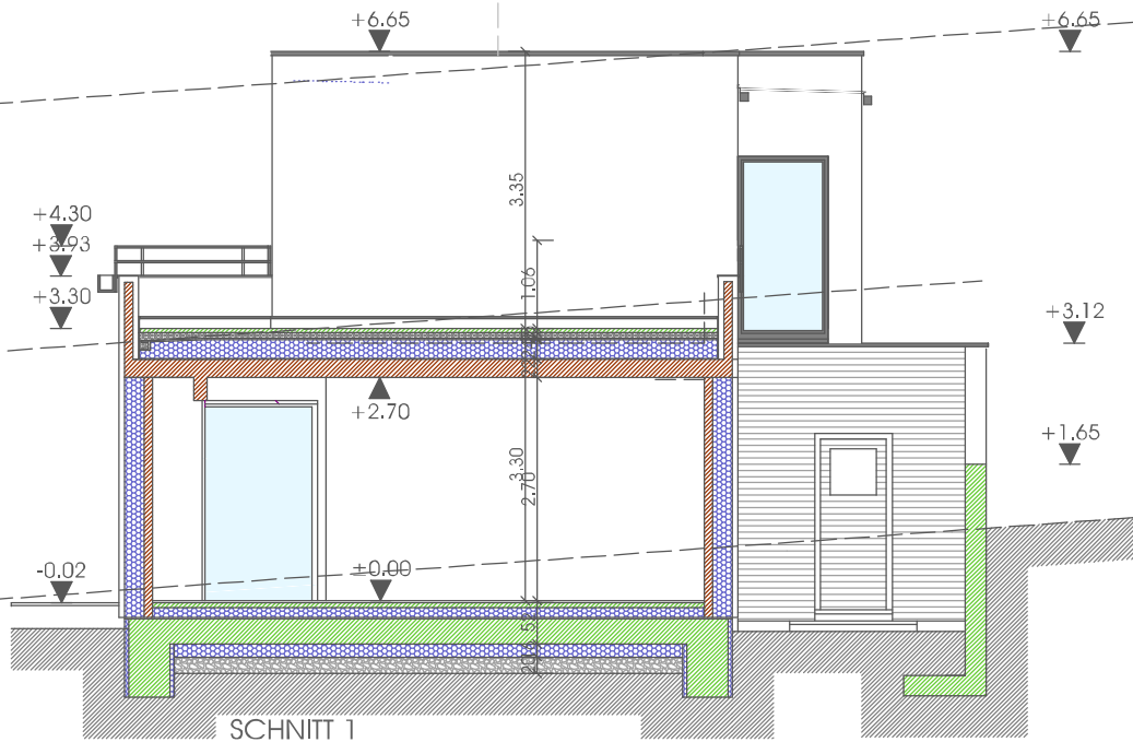
SCHNITT 1
